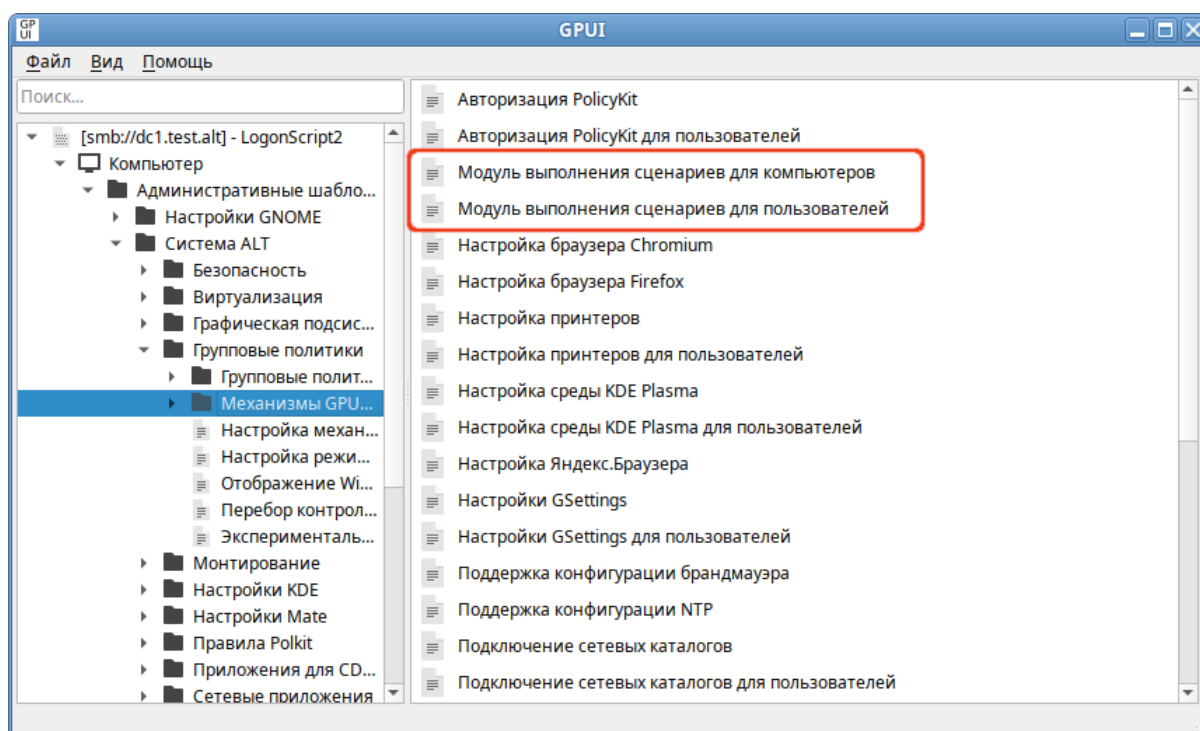
Рис. 235 – Механизмы GPOUpdate управления logon-скриптами
