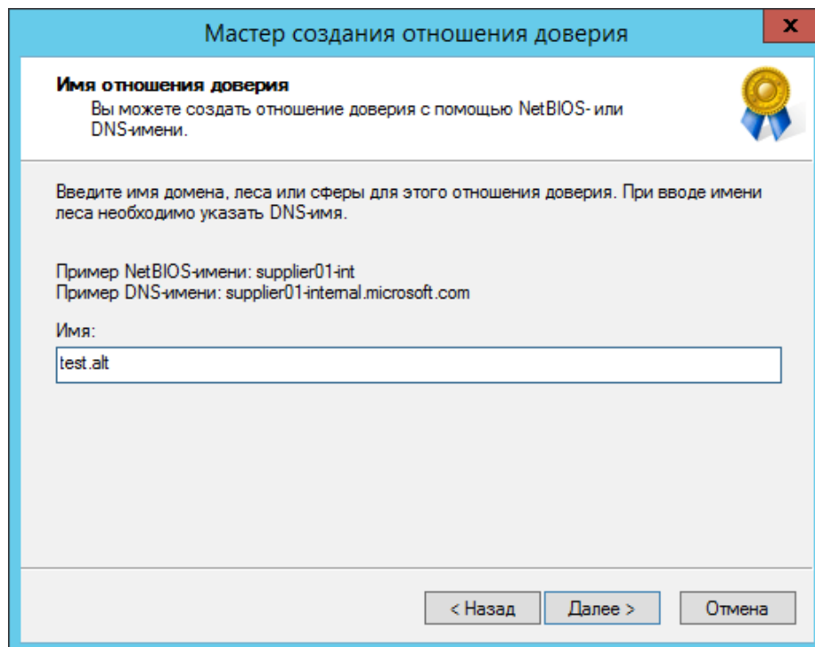
Рис. 256 – Окно ввода имени домена Samba DC
