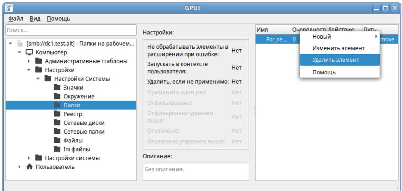
Рис. 162 – Контекстное меню элемента предпочтения
