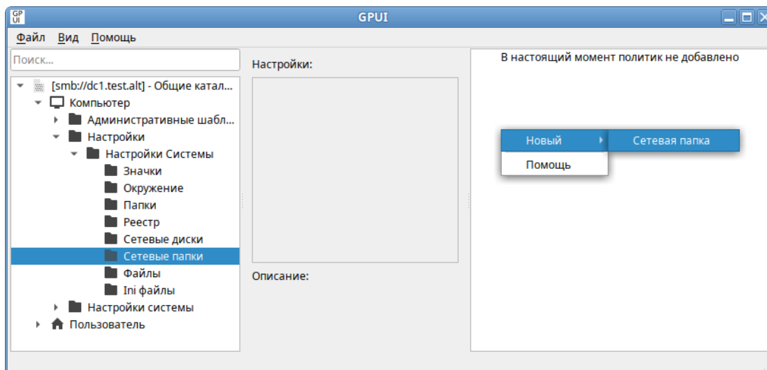
Рис. 216 – Создание новой политики «Сетевая папка»
