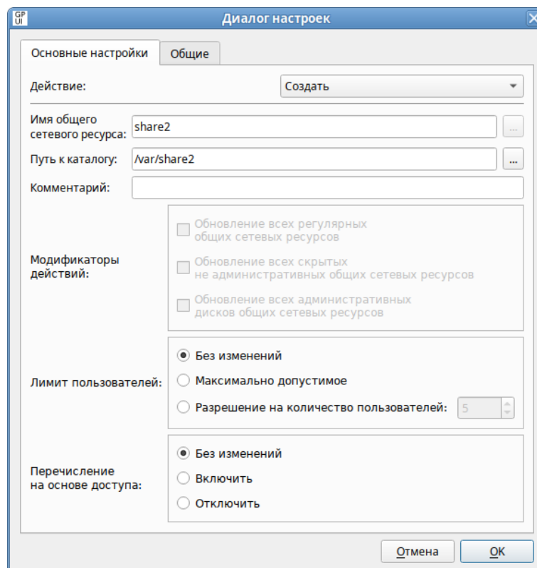
Рис. 217 – Настройки политики «Сетевая папка»
