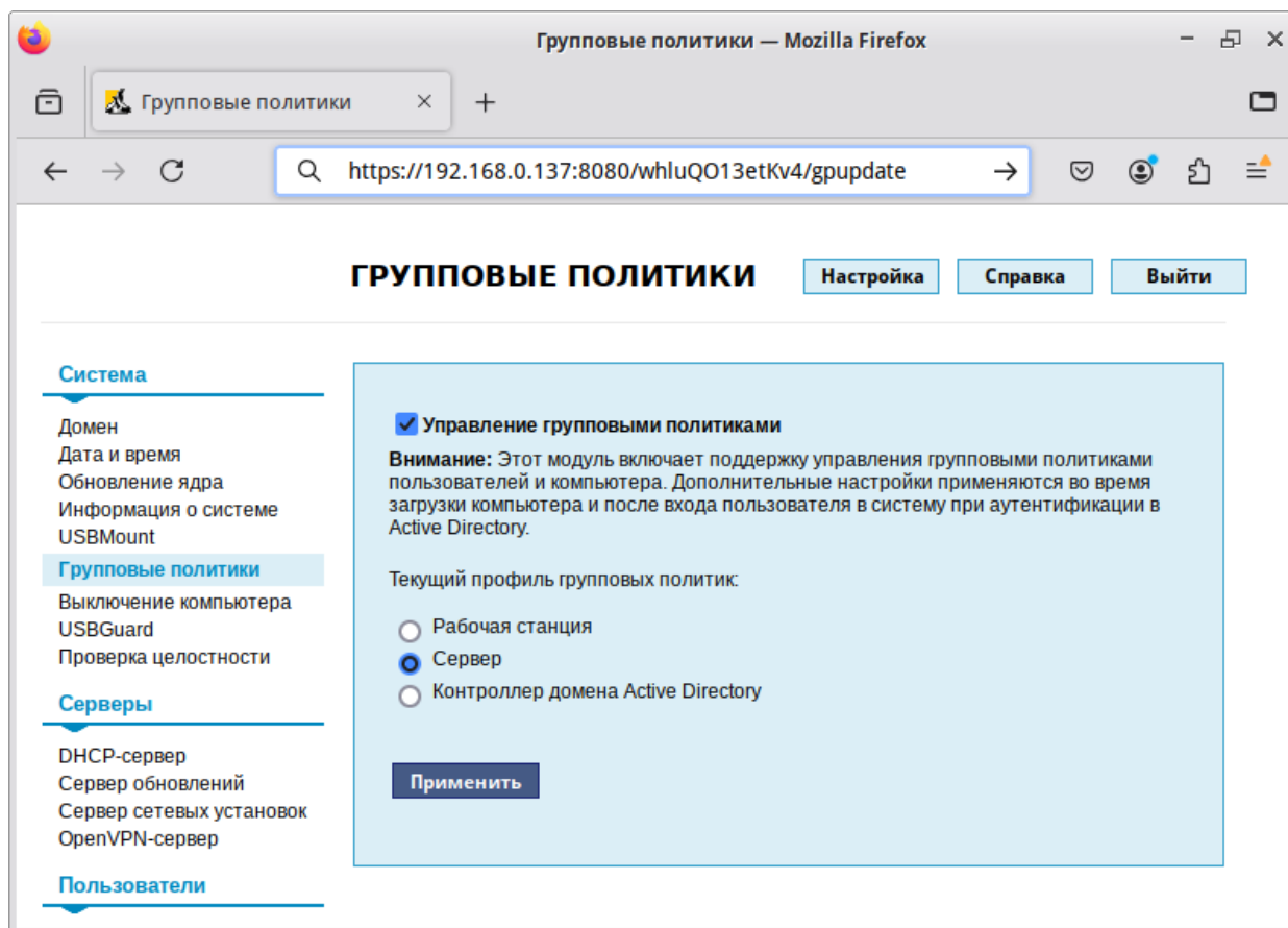
Рис. 38 – Веб-интерфейс модуля «Групповые политики»
