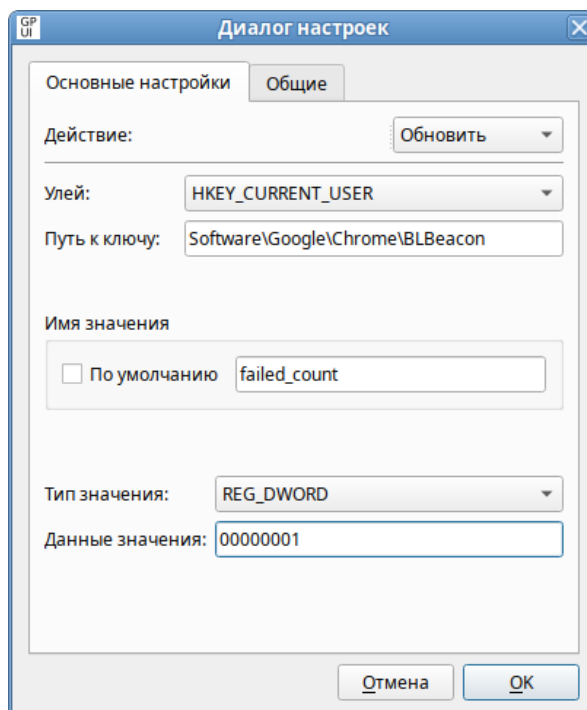
Рис. 225 – Настройки политики «Значение реестра»
