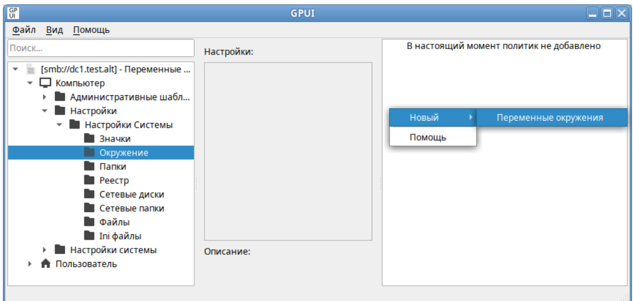
Рис. 207 – Новая политика «Переменные окружения»
