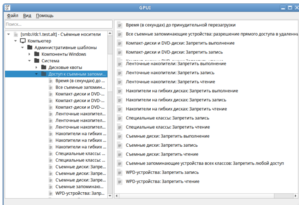
Рис. 175 – «Доступ к съемным запоминающим устройствам»
