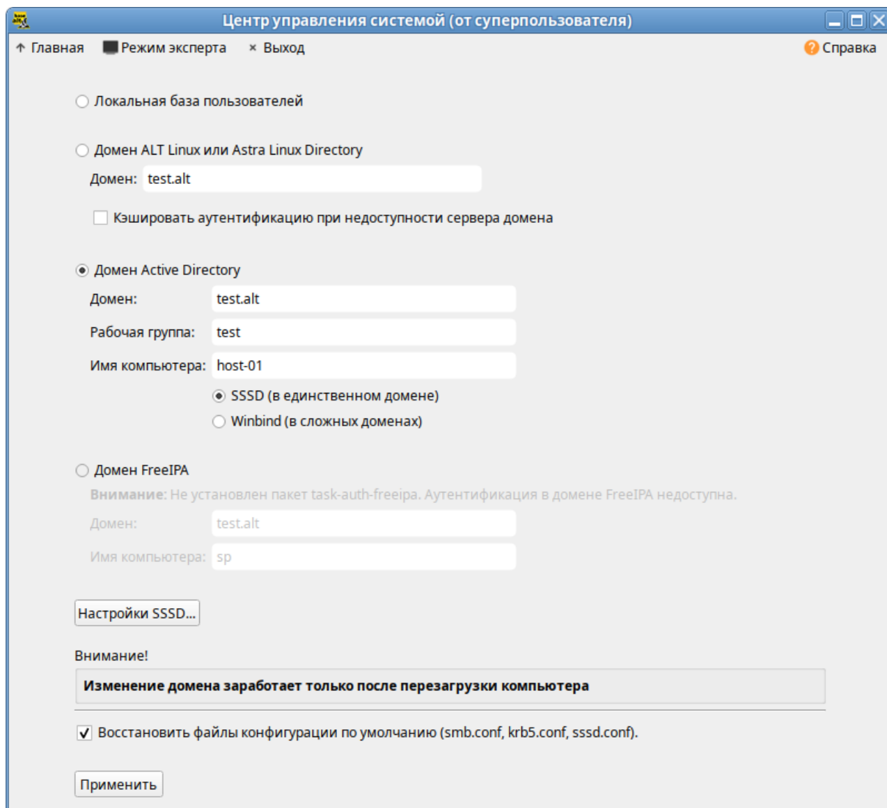
Рис. 23 – Ввод в домен в «Центр управления системой»
