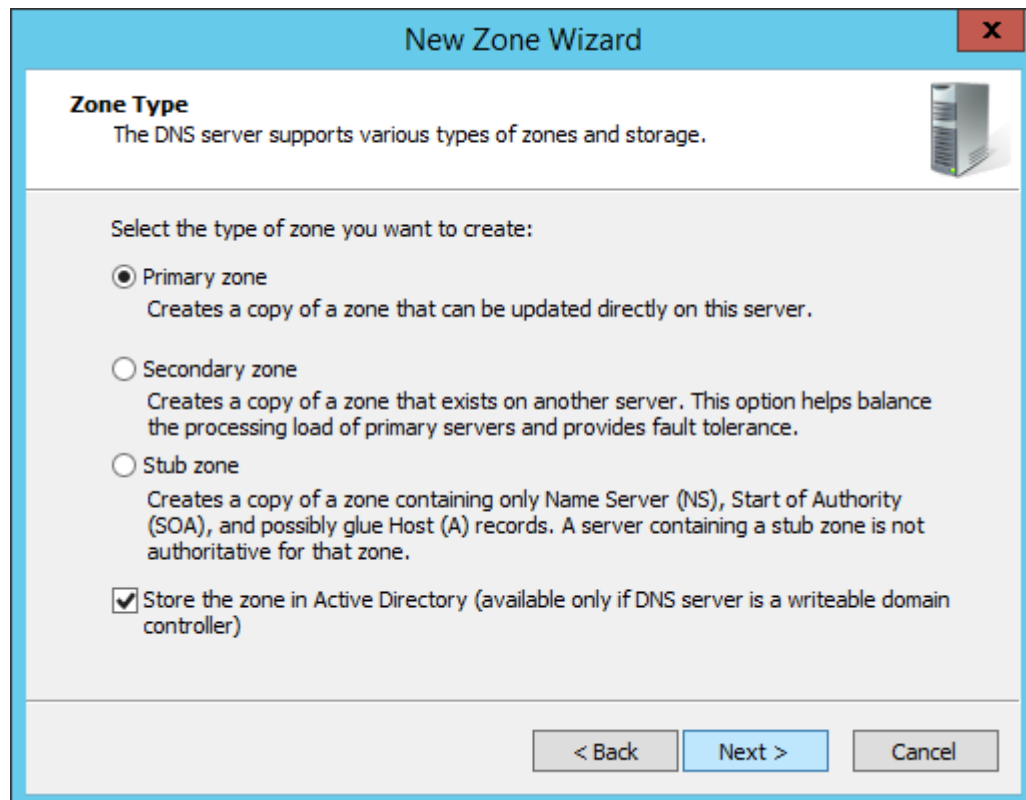
Рис. 281 – Выбор типа зоны
