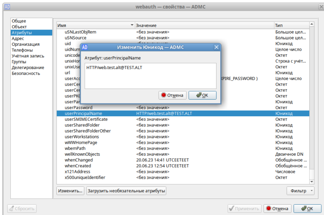
Рис. 289 – Изменение параметра userPrincipalName в ADMS
