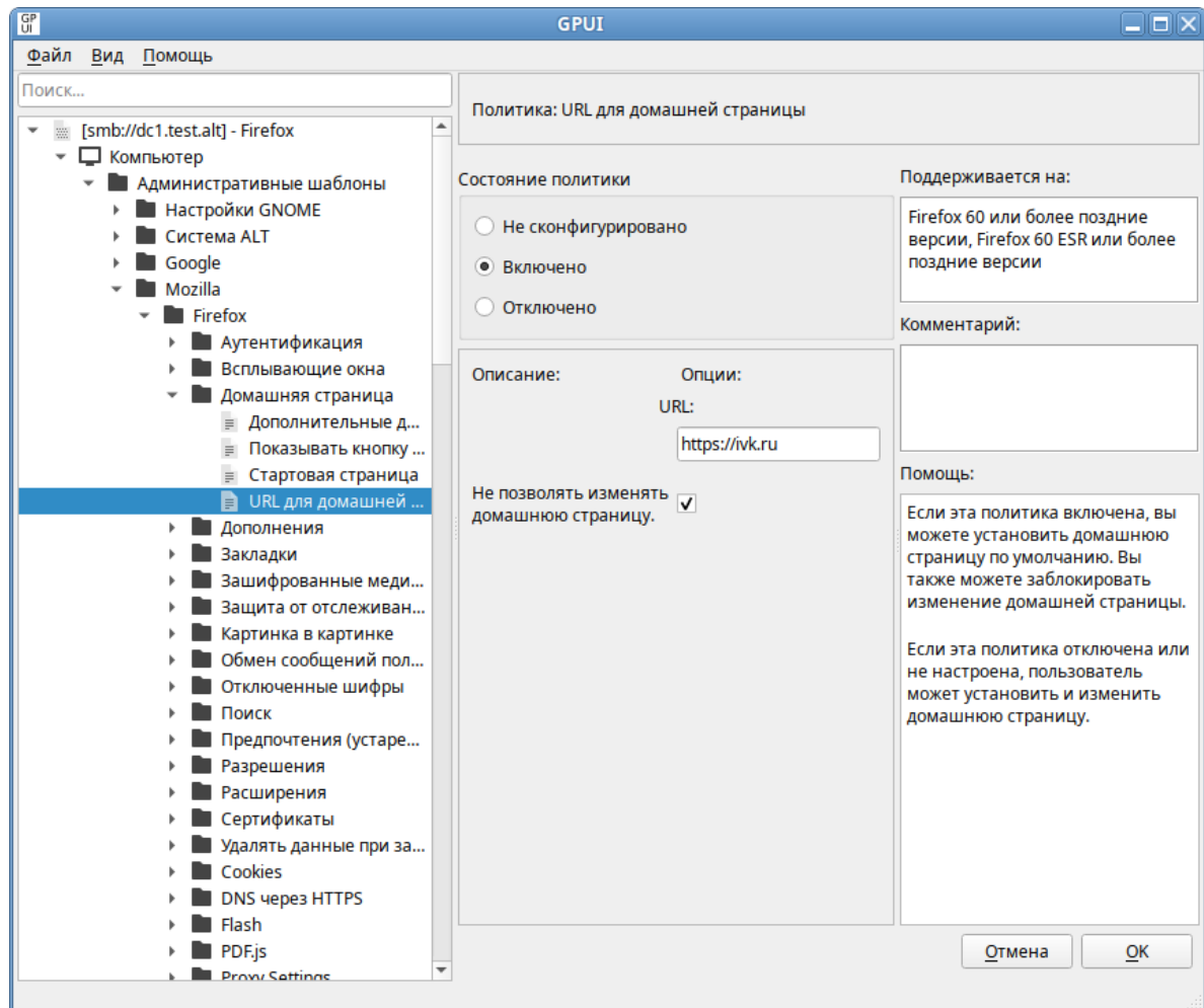
Рис. 192 – Диалоговое окно «URL для домашней страницы»
