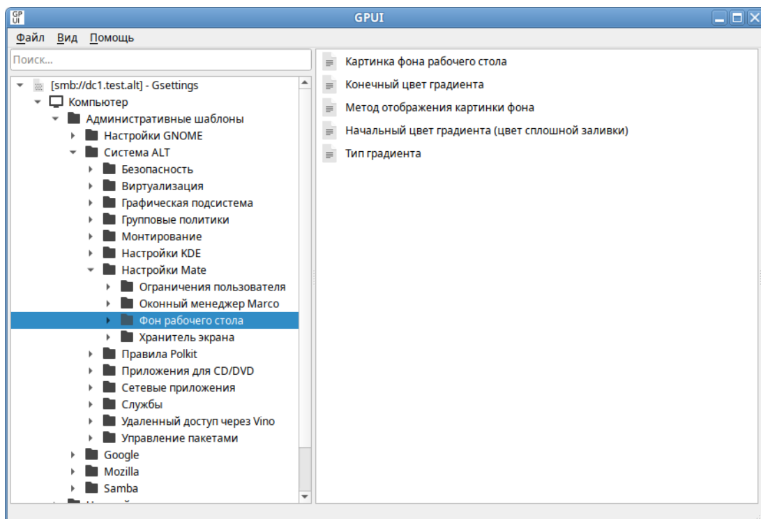
Рис. 177 – Управление настройками gsettings
