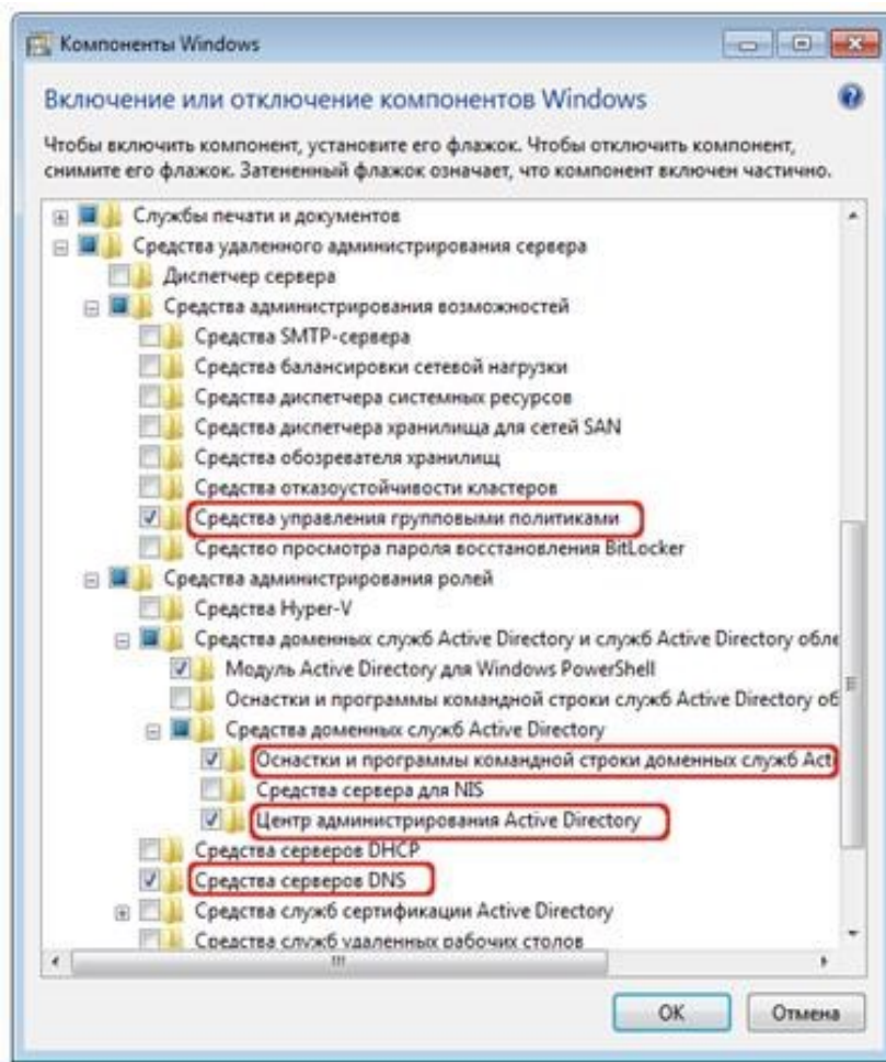
Рис. 34 – Компоненты для включения
