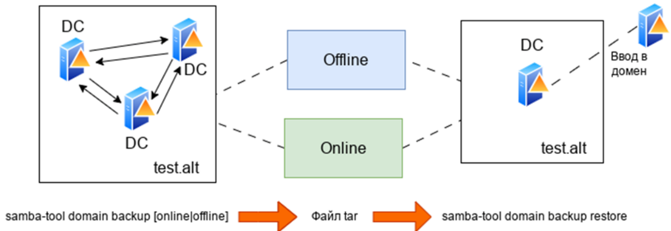
Рис. 287 – Схема создания резервной копии
